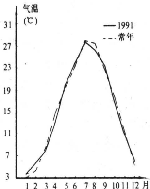
1991年及常年各月平均气温
