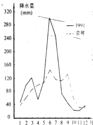
1991年及常年各月降水量
