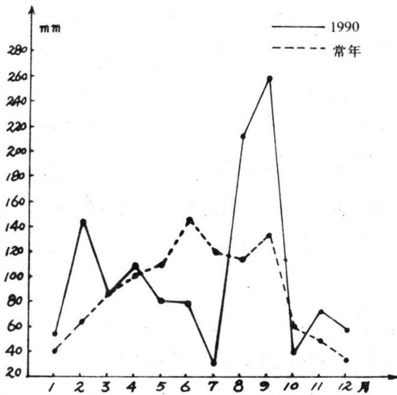
图三: 吴江县气象站 1990 年及常年各月降水量
