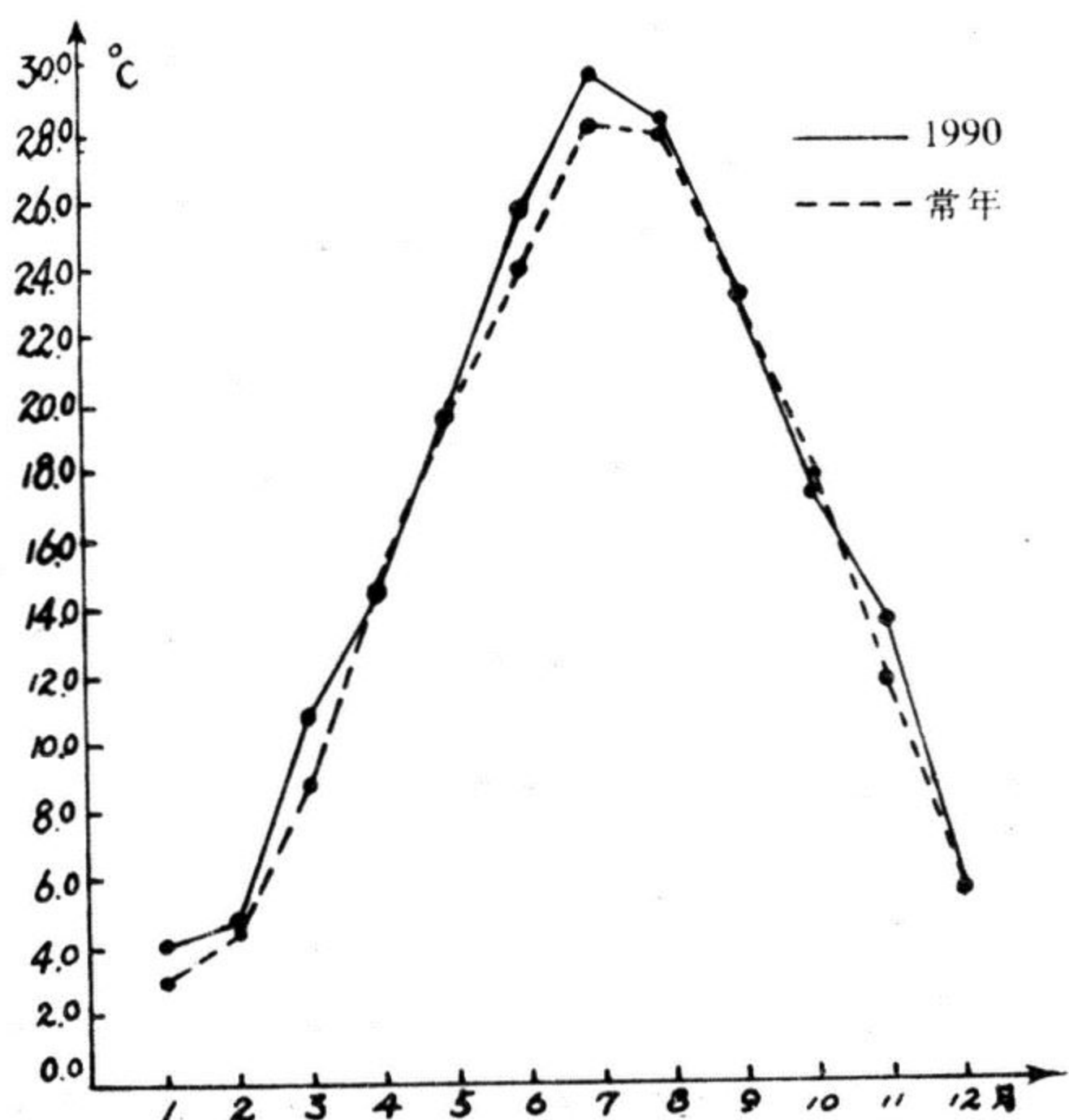
图一：吴江县气象站 1990 年及常年各月平均气温
