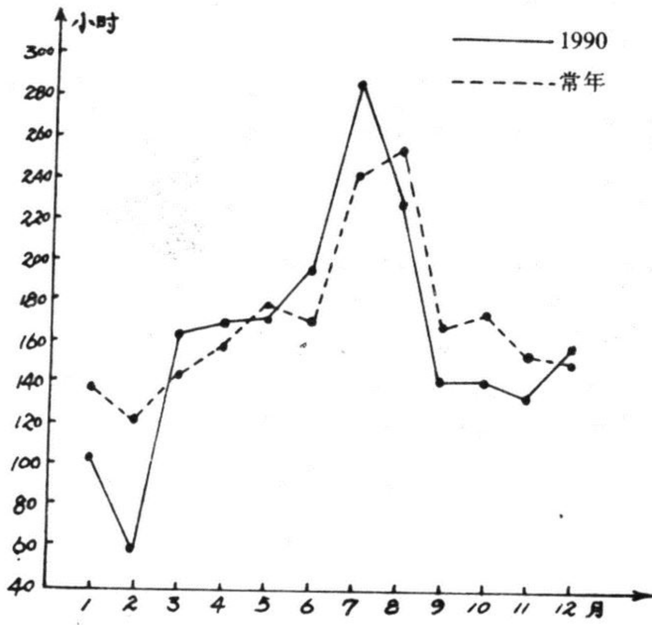
图二: 吴江气象站 1990 年及常年各月日照时数
